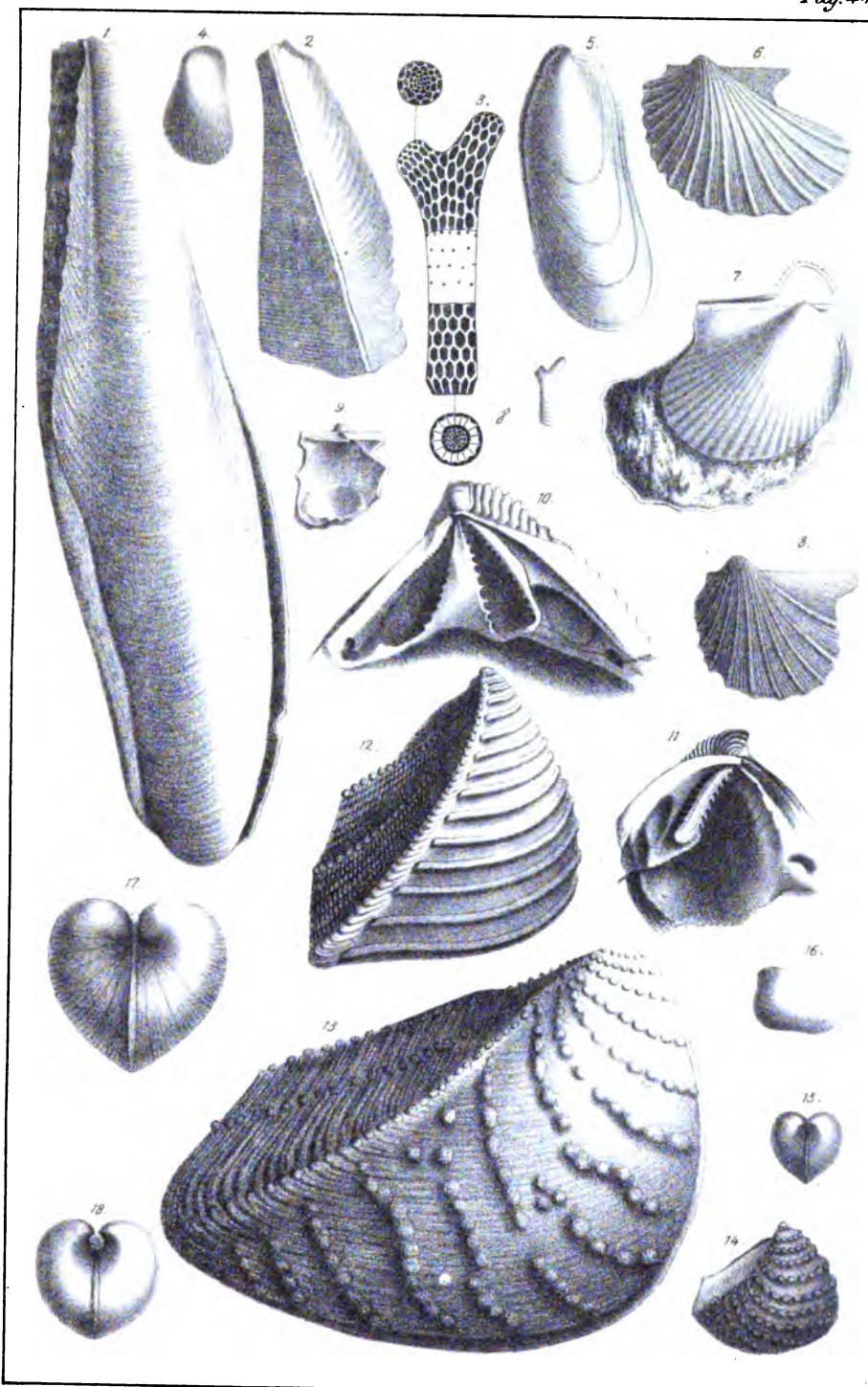
Quenstedt Jura.
